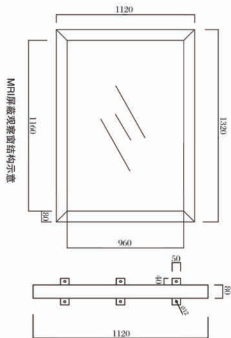
MRI屏蔽观察窗结构示意图
