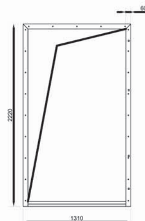
Door Frame
